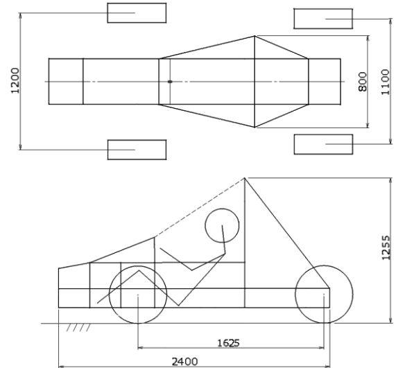
図 5 3D-CAD による 2D ジオメトリーの設計 (図中では主な寸法のみ記載)
